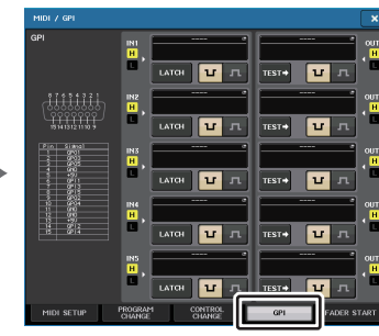
MIDI/GPI 画面
