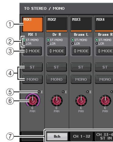
ST/MONO モード
